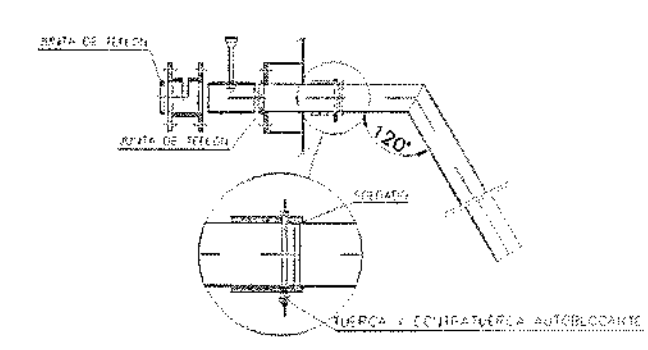
DETALLE COUDE DECANTEUR DETALLE CODO DECANADOR
