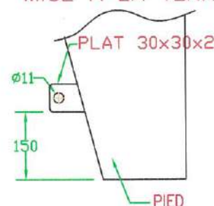
DETAIL C4: PATTE DE MISE A LA TERRE
